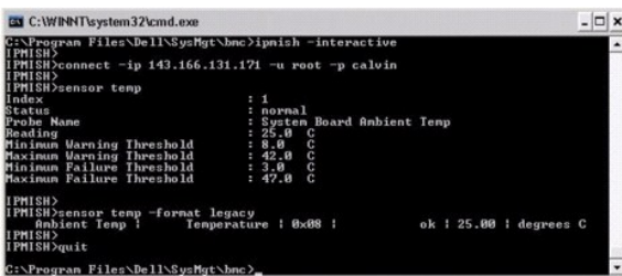
Figure 3-12. Exemple d'option de capteur
