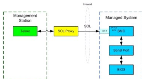
Figure 3-15. Diagramme du serveur proxy SOL
